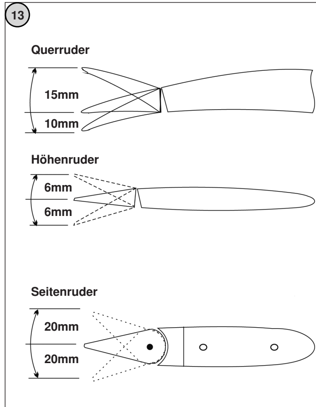
Bild 13 Ruderausschläge
