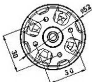
(Unit單位:mm)
