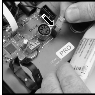
Abb. 9.4.4.2.: Akku anschließen
