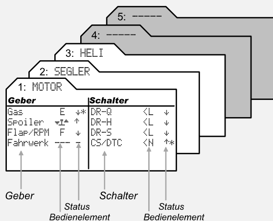
Abb. 11.3.5.1.: globale Zuordnungslisten
