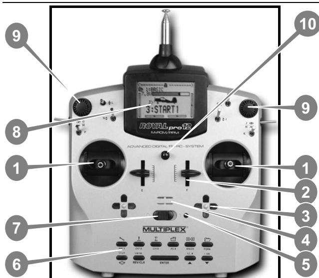
Abb. 9.1.1.: Senderoberseite (Schalter K und P nachgerüstet. Nicht im Lieferumfang!)
