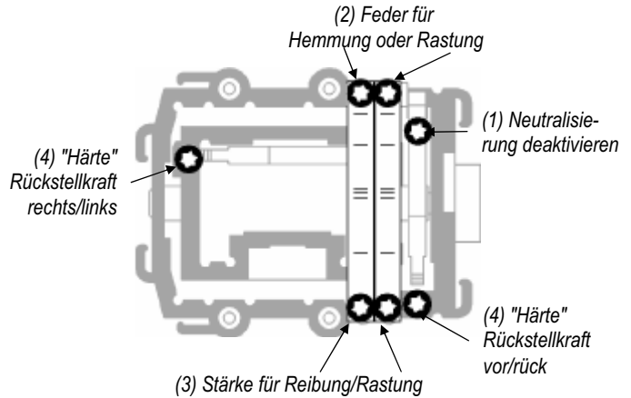
Abb. 9.4.5.1.: Einstellschrauben am Knüppel
